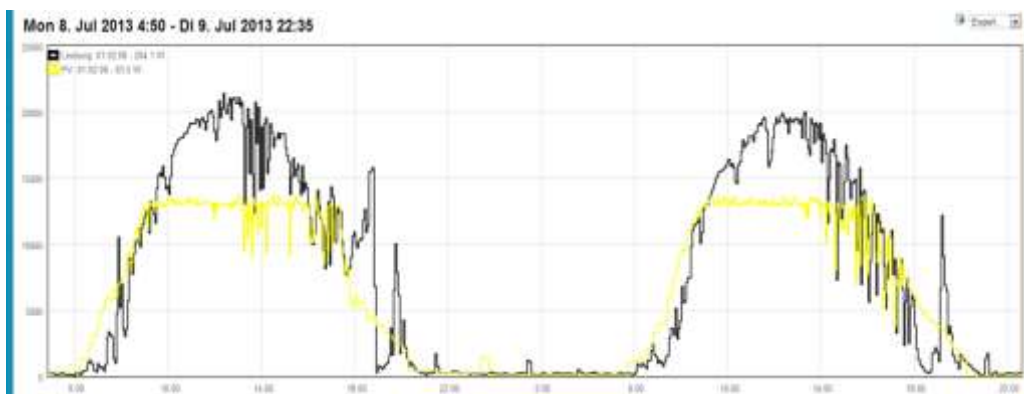
Bild 2: Impulszählung mit alter Version s0vz. Es können nicht mehr als 12500 Impulse gezählt werden.
